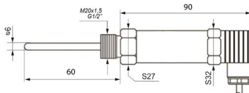
Рисунок 1 – Термопреобразователь с цифровым выходом T.Pt – RS – DIN – 6 – 60 – (-70/+200)
